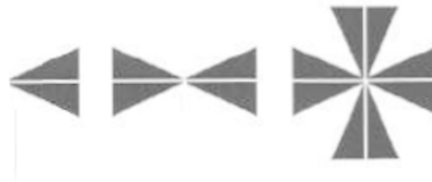
Fig. 8. Dn motifs symmetry
